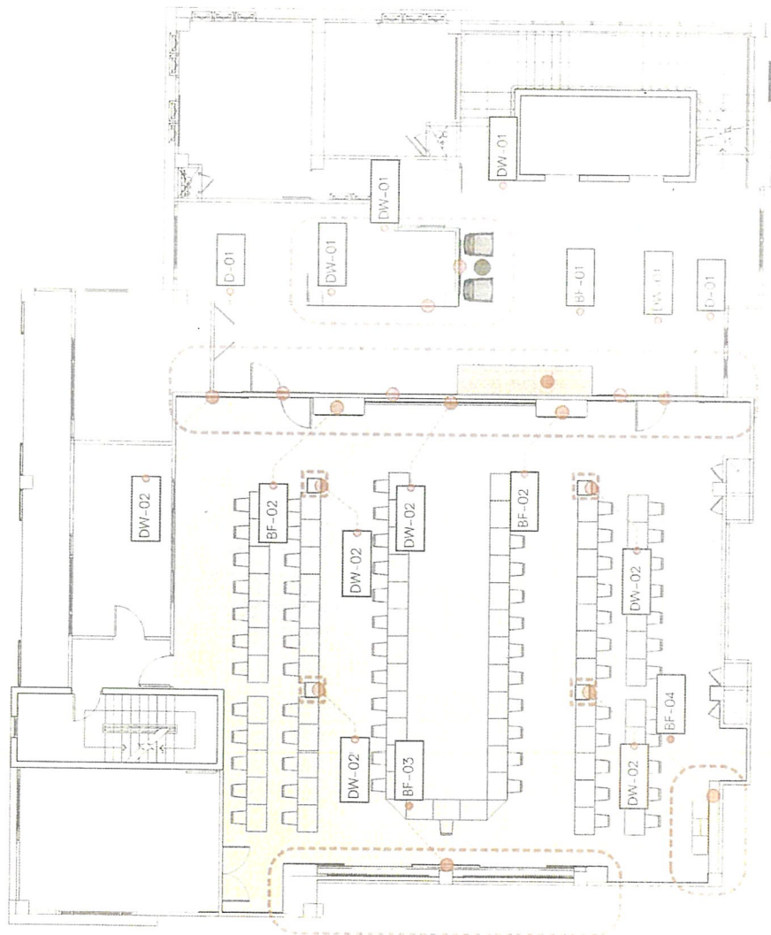
ห้องประชุมชั้น 5 อาคารสำนักงานอธิการบดี มาตราส่วน 1 : 125
